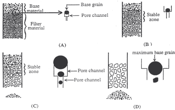
Figure 1 – Les différents cas de rétention particulaire à l'interface entre deux couches [9]
